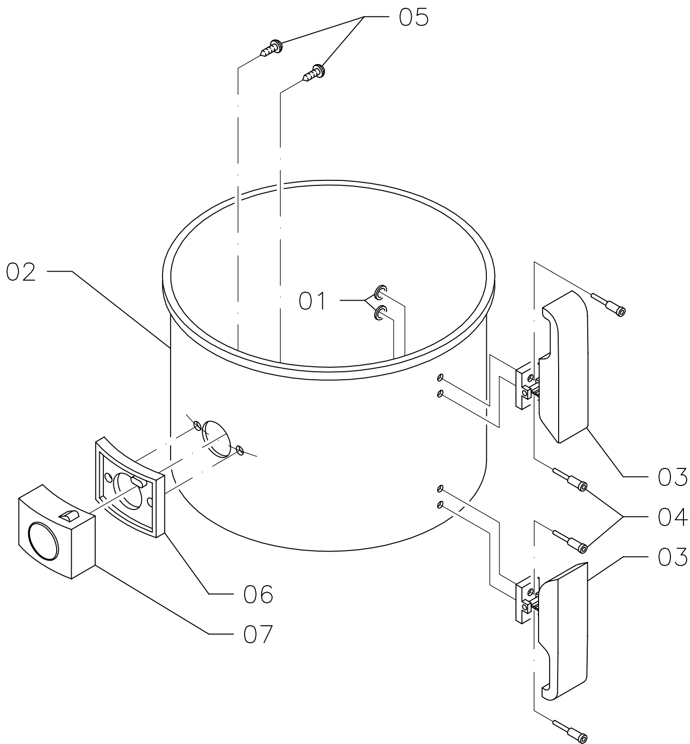
FUSTO H230 COMPLETO 4GANCI COD. FS8000 REALIZZATO DA U.T. IL 09/01/2004 REV.1
